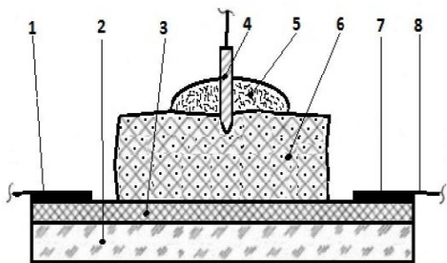
Рис. 5. Эскиз устройства PPC-OECT 1. Контакт истока, углеродная паста, 2. Подложка, стекло, 3. Полупроводник, PEDOT:PSS), 4. Затвор, Ag, 5. Капля раствора PPC, 6. Мембрана, PDMS, 7. Контакт стока, углеродная паста, 8. Проволока. (Составлен на основе описания и фотографии в статье [38,]).
